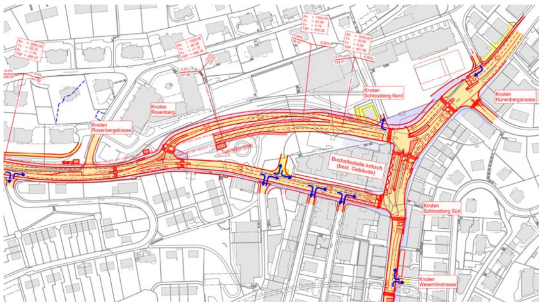
Abb. 41: Tunnel Rosenberg mit Anschluss Schlossberg Nord
